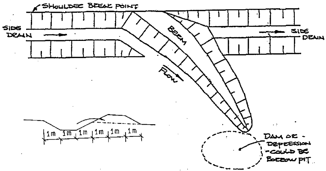
MITRE DRAIN DETAILS
